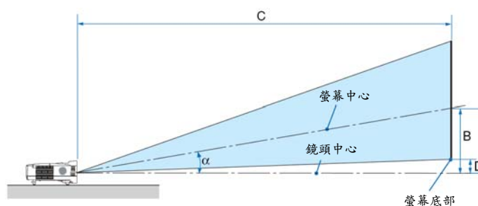
距離圖[NP610S/NP510WS]
