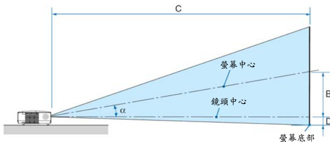
距離圖[NP610/NP510/NP410/NP405/NP310/NP305/NP510W/NP410W]
